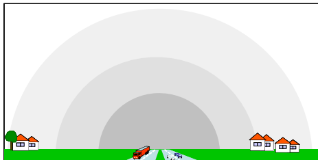
Fig. 8a L'inquinante emesso in aree di pianura può disperdersi in tutto il semispazio che sovrasta la superficie del terreno. Le tonalità di grigio del disegno indicano qui le aumentate concentrazioni medie sempre per una distribuzione uniforme di direzioni del vento.
