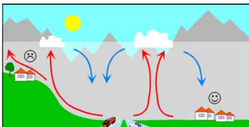
Fig. 11a Venti di pendio (rossi a sinistra) e termiche (rosse a destra) portano durante il giorno a sviluppare uno spesso strato rimescolato. Questo riduce le concentrazioni sul fondovalle ma trasporta gli inquinanti lungo i pendii. Correnti di compensazione sono indicate in blu.
