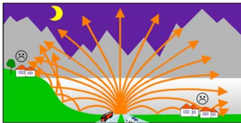
Fig. 12b Direzione di dispersione dei raggi sonori durante la notte quando la temperatura dell'aria aumenta con la quota in uno strato d'inversione (in grigio) e il suono è rifratto verso il basso. Non compaiono zone acusticamente in ombra e il suono è riflesso al suolo.
