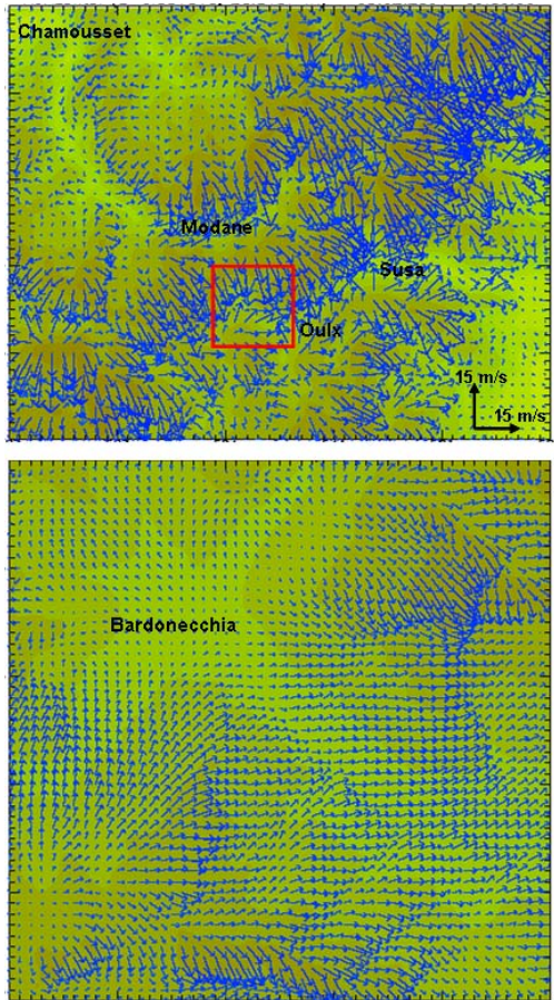
Fig. 19 Esempio di simulazioni meteorologiche "in-nestate" del campo di vento con 1 km di risoluzione (in alto) e in un sottodomino (riquadro rosso) con 100 m di risoluzione (in basso).
