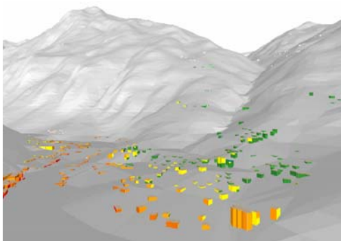
Fig. 21 Esempio di mappe di rumore. I colori rappresentano i livelli di rumore simulati sulle facciate degli edifici della Val Maurienne in Francia. Tonalità dal verde al rosso indicano livelli crescenti.
