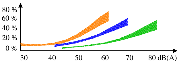
Fig. 14 Esempio di una funzione esposizione-risposta che mostra la porzione di popolazione "molto infastidita" in funzione dei livelli sonori di lungo termine per il rumore di una strada principale (in rosso), un'autostrada (in blu) e una ferrovia (in verde).
