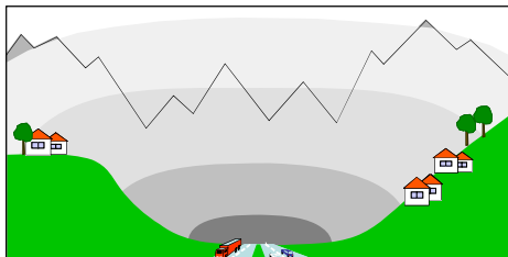
Fig. 8b In una valle il volume d'aria è ridotto per la presenza dei pendii. Le tonalità di grigio del disegno indicano qui le aumentate concentrazioni medie sempre per una distribuzione uniforme di direzioni del vento
