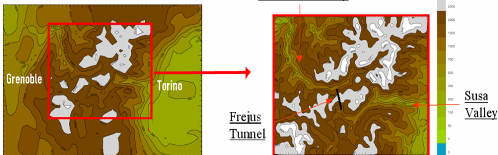
Fig. 18 Effetto della risoluzione spaziale: il grafico mostra l'elevazione del terreno delle Alpi occidentali con una risoluzione spaziale di 4 km (a sinistra). Nel sottodominio evidenziato (riquadro rosso) la risoluzione spaziale è portata ad 1 km (a destra) rendendo visibili molti più dettagli dell'orografia.
