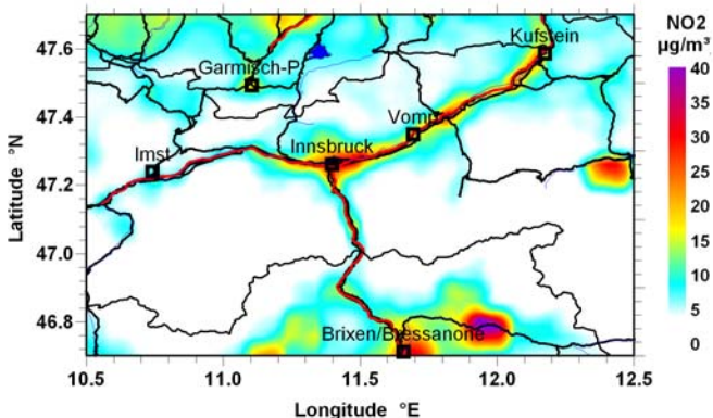
Fig 20 Esempio di simulazione della concentrazione media annuale di \text{NO}_2 in una vasta area delle Alpi orientali.
