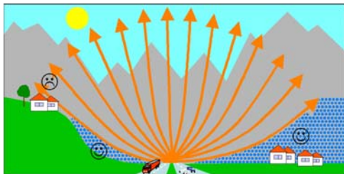
Fig. 12a Direzione di dispersione dei raggi sonori durante il giorno quando la temperatura dell'aria decresce con la quota e il suono è rifratto verso l'alto. Nelle aree punteggiate in blu ("zone "acusticamente in ombra") del fondovalle il rumore è marcatamente ridotto poiché i raggi sonori rifratti verso l'alto non le possono raggiungere.
