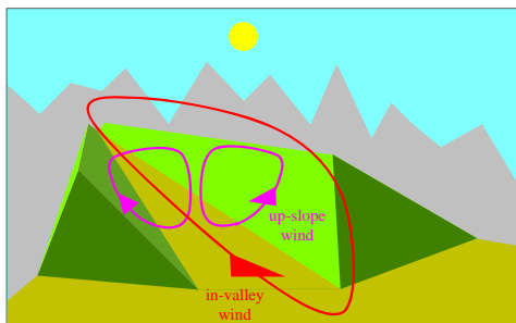
Fig. 6a Nel primo pomeriggio di giornate serene si sviluppano venti che risalgono i pendii (magenta) e circolazioni che penetrano nelle valli (rosso).
